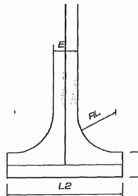
AIRE DERETOURNEMENT «CE T» E= 5,00m RL= 0,00m L2=24,00m
