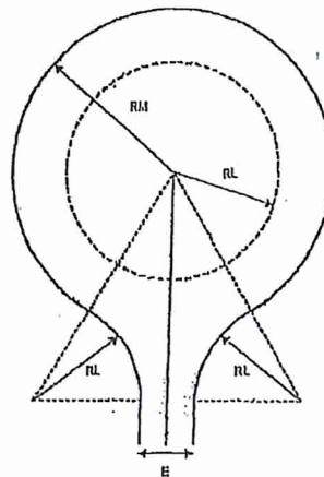
AIRE DERETOURNEMENT «EN L» E= 4,00m RL= 0,00m RM=13,00m
