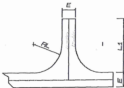
AIRE DERETOURNEMENT «ENL» E= 4,00m RL= 0,00m L1=15,00m L'=13,00m
